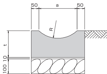
基礎一体型
