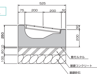
参考重量：112kg(L=0.6m) ※グレーチングの重量は含まない。
