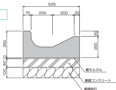
参考重量：115kg (L=0.6m)
