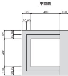
製品図
