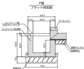
設置図
