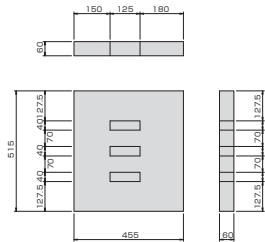
街渠枡用蓋
