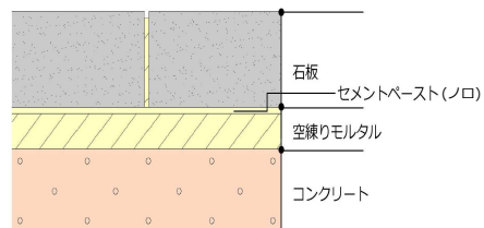
参考断面図
