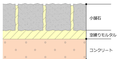
参考断面図
