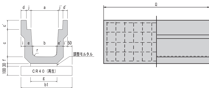
寸法表
