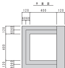
プレキャスト街渠枡単体図
