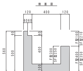
プレキャスト街渠枡設置図
