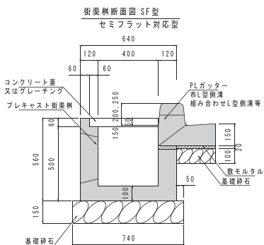
プレキャスト街渠枡設置図
