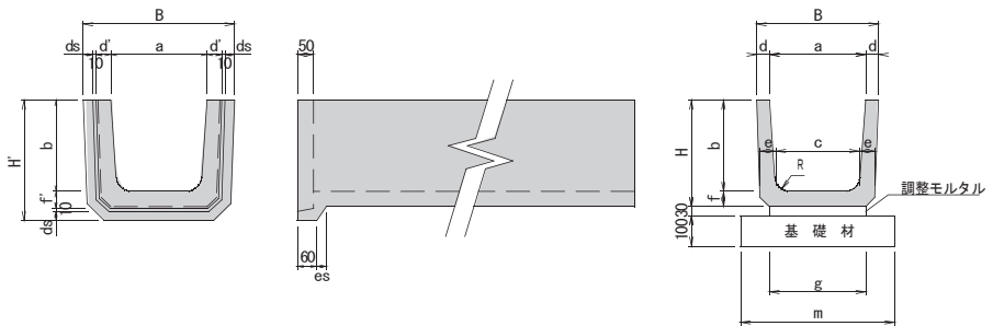
規格寸法図
