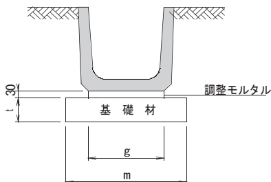
標準施工断面図
